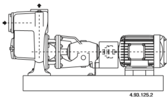
Obr.4 Vyrovnání spojky
