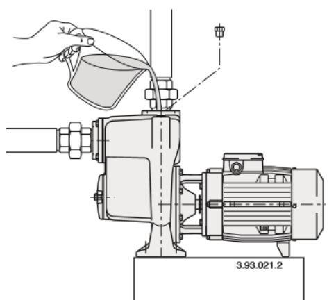
Obr.2 Plnění
