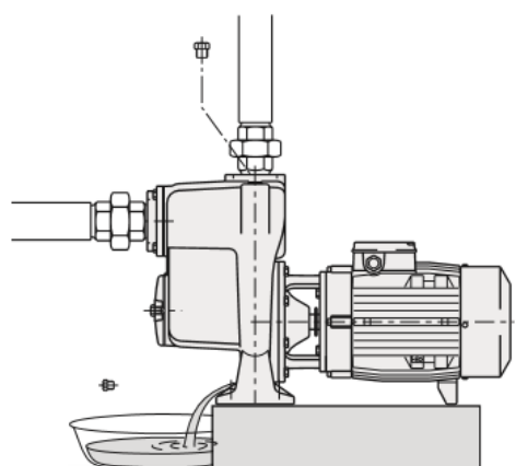
Obr.3 Vypouštění
